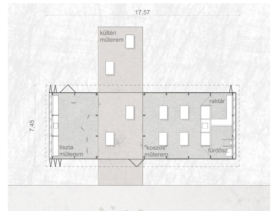
műhely homlokzata, alaprajza 1:200
