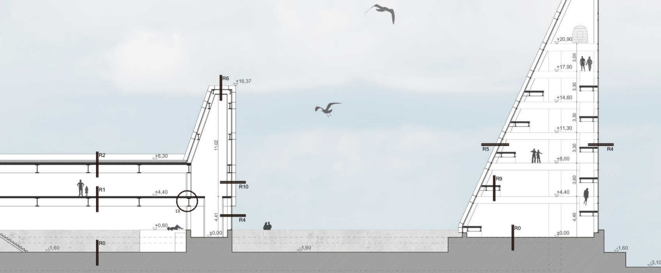
A-A METSZET M1:250
