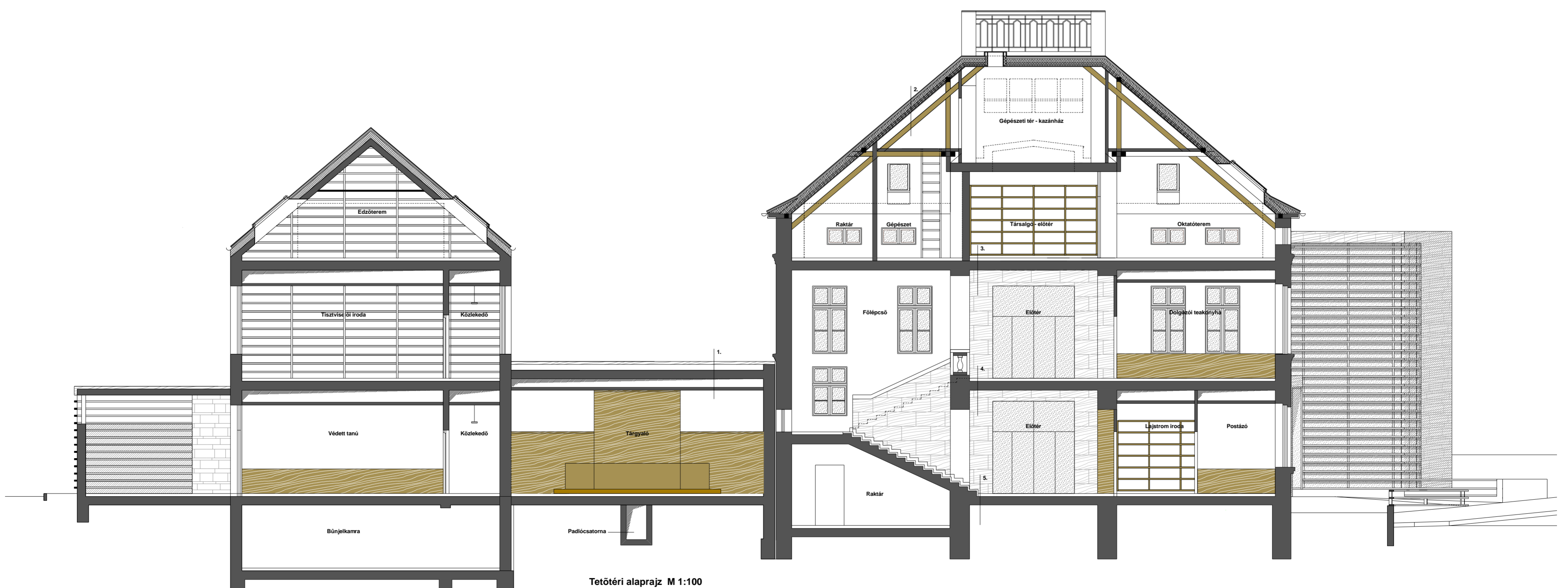
Tetőtéri alaprajz M 1:100
