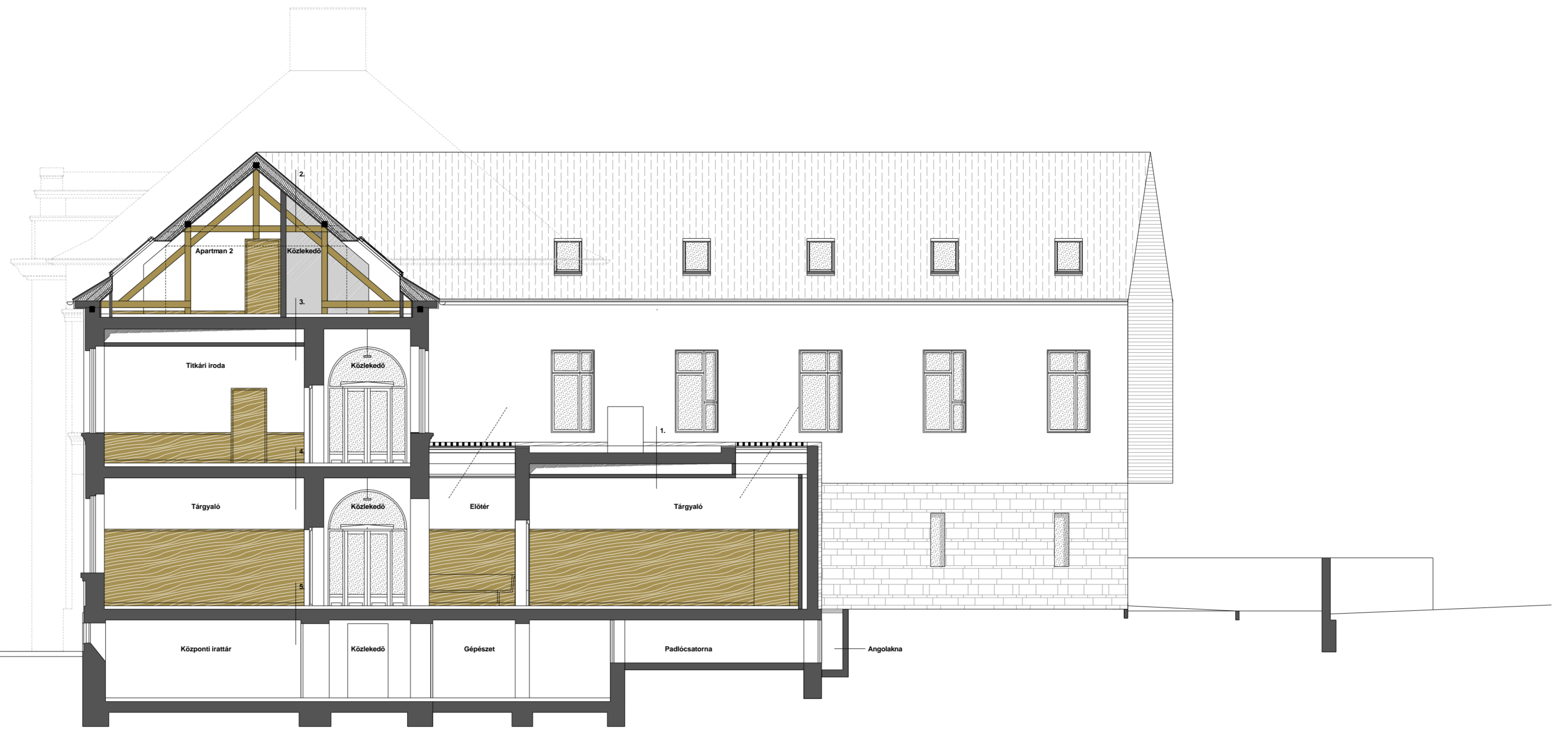
A-A Metszet M 1:100
