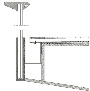
Gyaloghíd részletrajza
