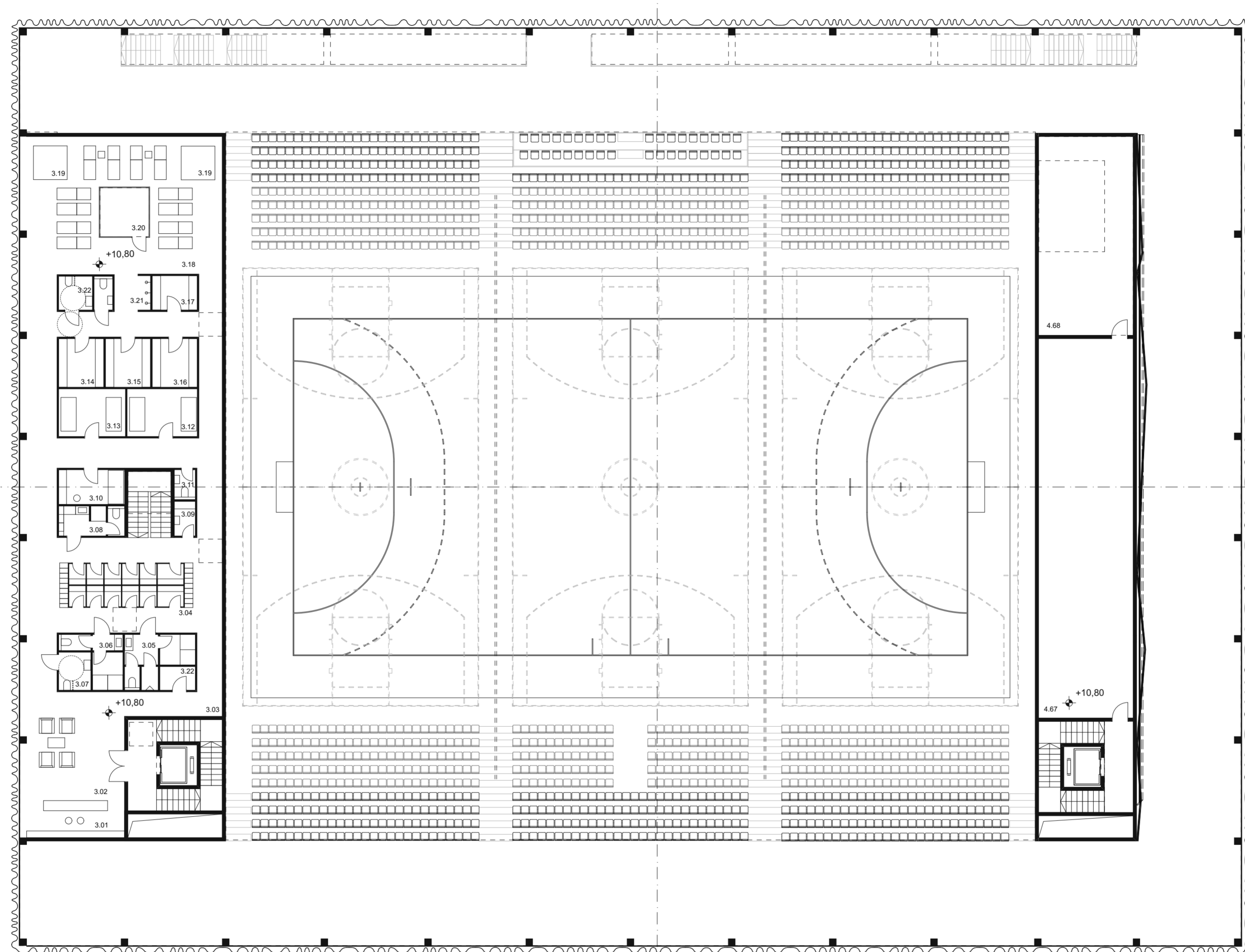
Harmadik Emeleti Alaprajz M 1:200
