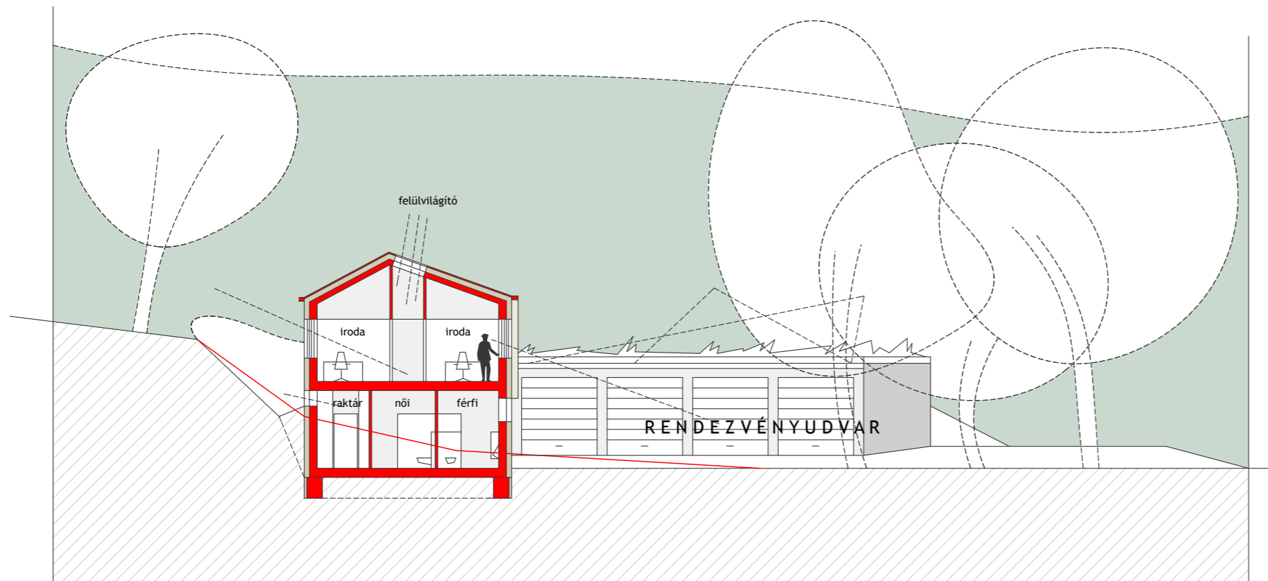
A-A METSZET
