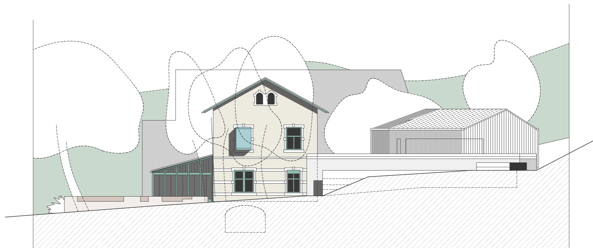
ÉSZAKI HOMLOKZAT _ MEGÉRKEZÉS FELŐL
