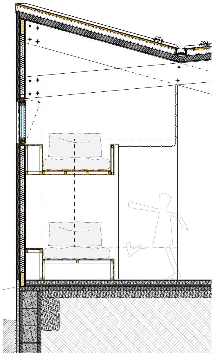
KERESZTMETSZET
