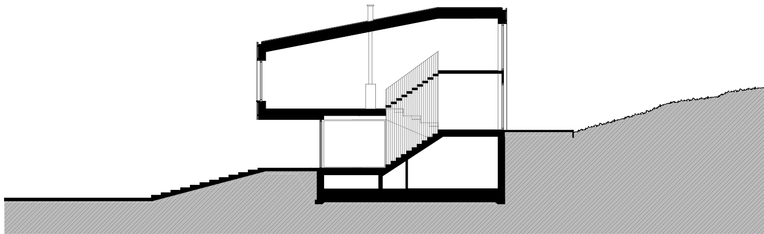
1-1 METSZET
