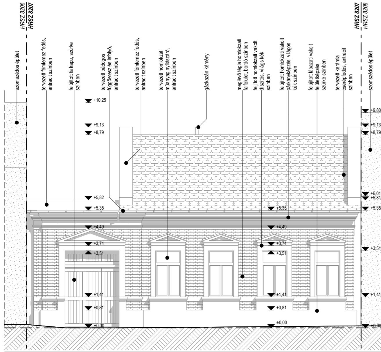
1. Homlokzat M=1:100
