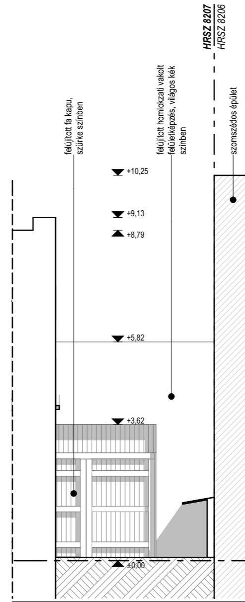
2. Homlokzat M=1:100
