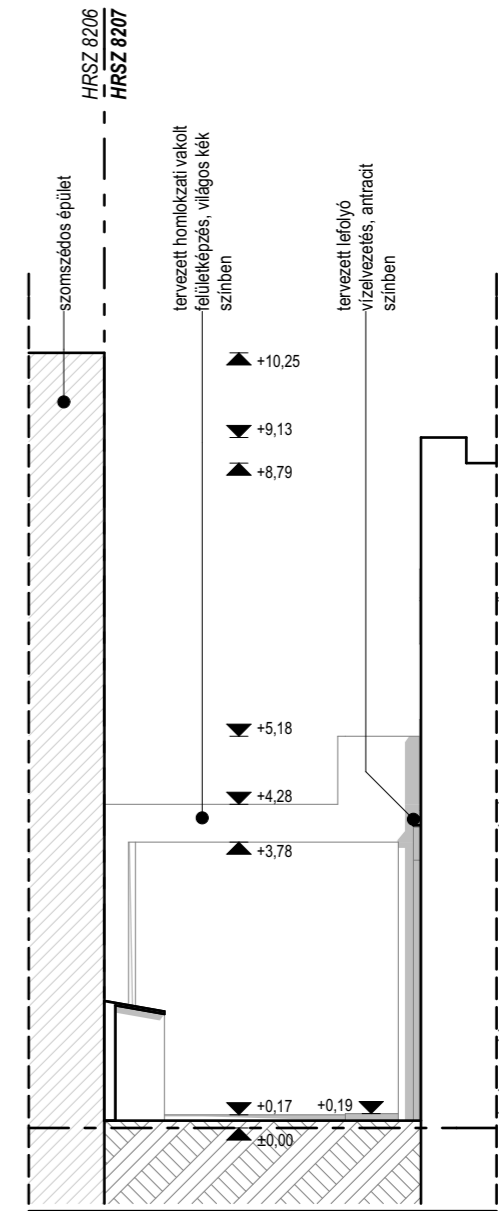
3. Homlokzat M=1:100
