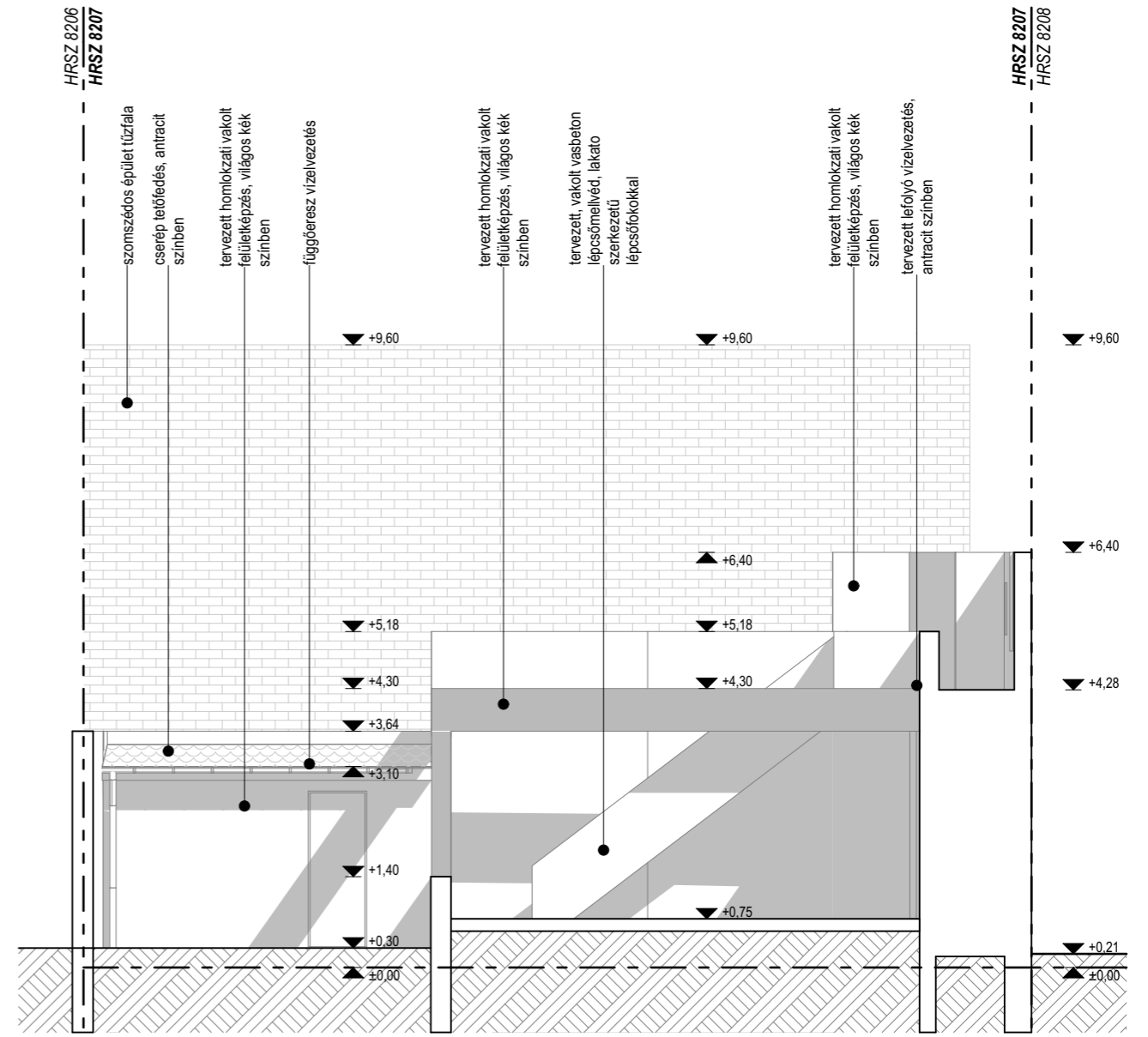
7. Homlokzat M=1:100
