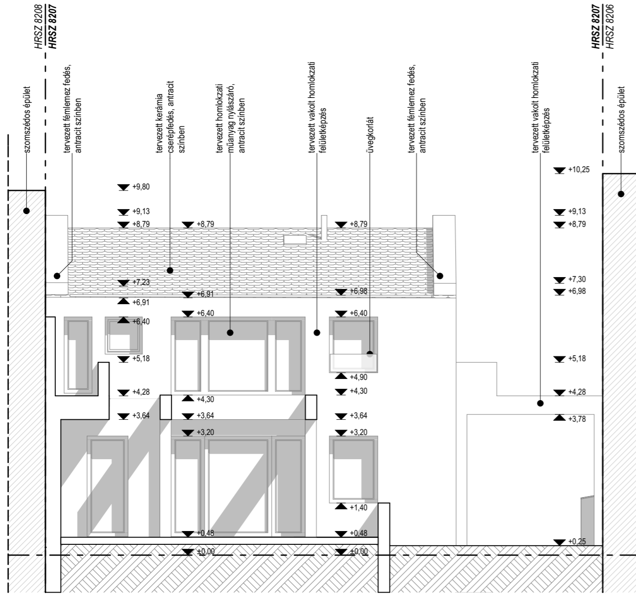
5. Homlokzat M=1:100
