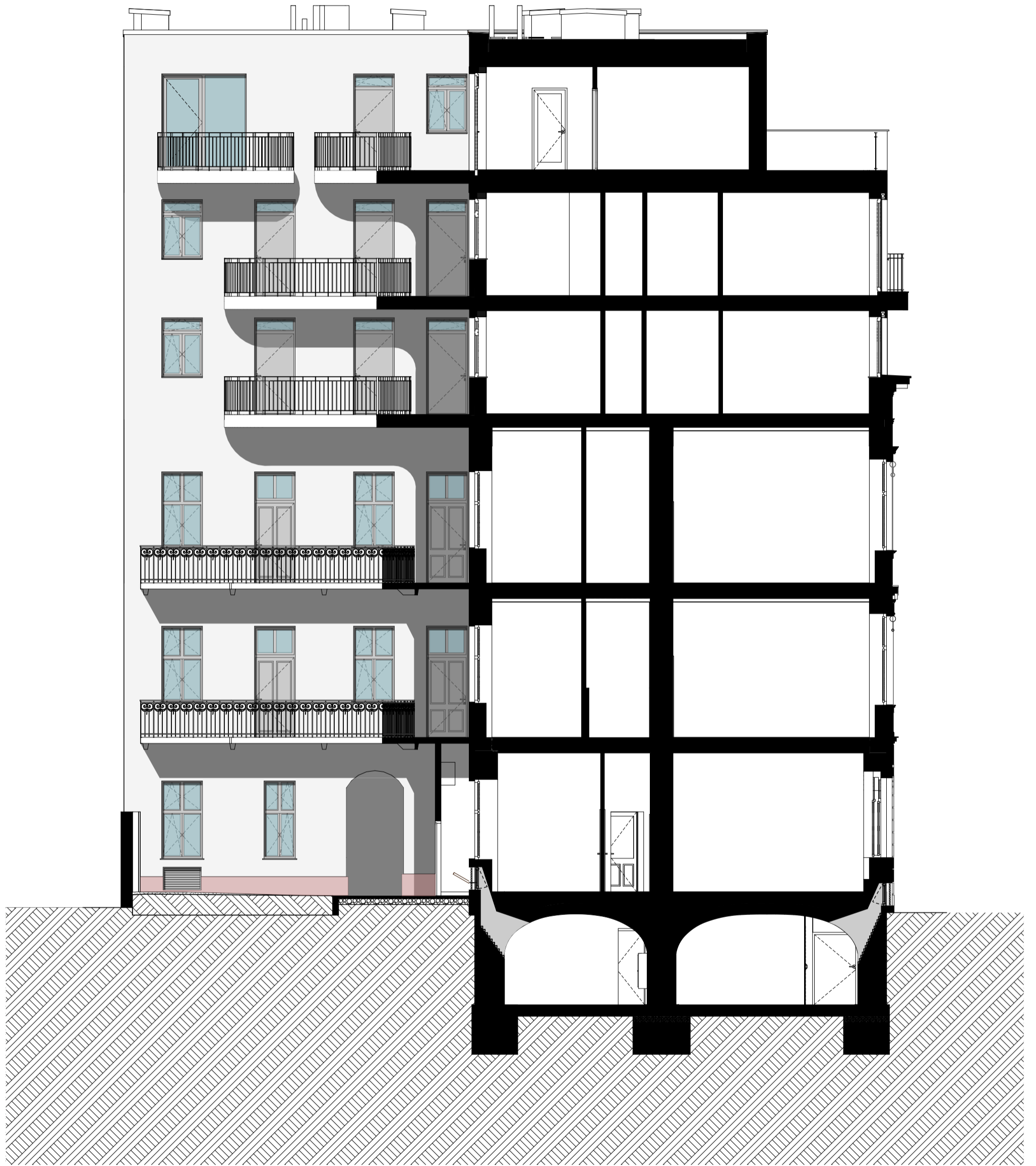
A-A metszet
