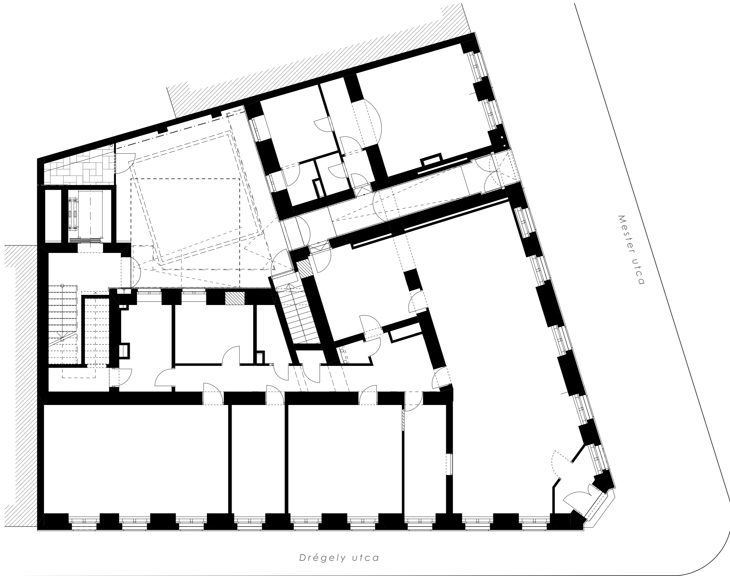
Földszinti alaprajz
